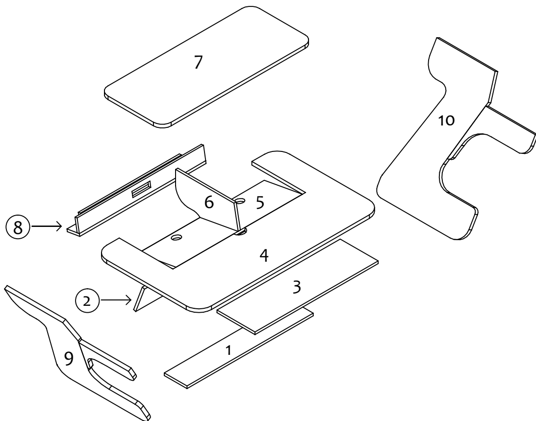
Part n° 2 Back stabilising bar
